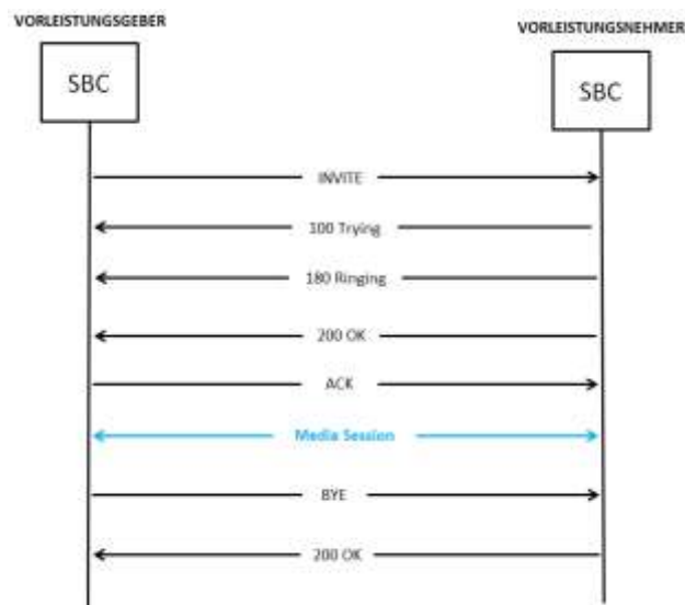
Abbildung 2 - Beispiel SIP Session (SBC – Session Border Controller)
